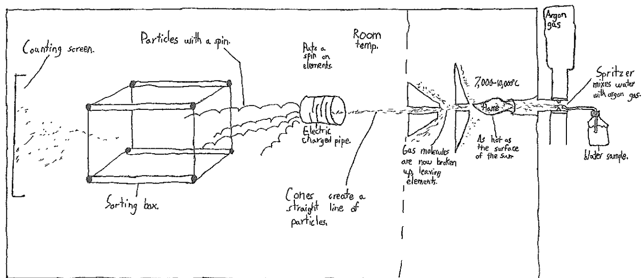
ICP-MS Diagram
